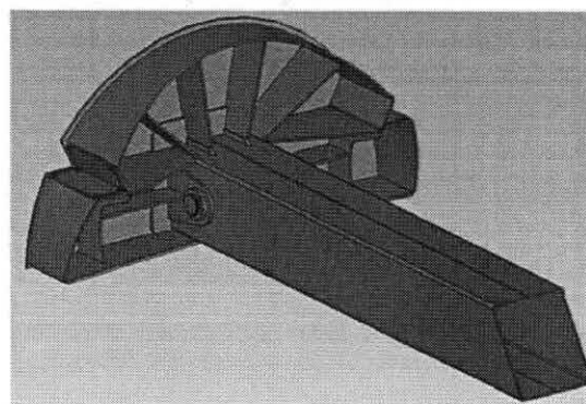
Modelado en 3D de la placa superior, utilizado para su construcción
