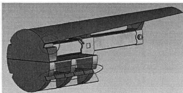
Modelado en 3D de la placa compactadora completa, utilizado para su construcción
