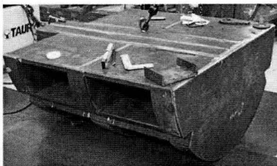
Parte inferior de la placa de compactación en proceso de fabricación.
